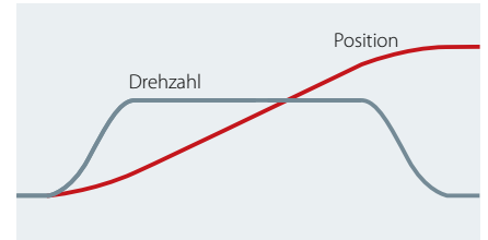
Abb. 2. Bewegungsprofil mit S-Rampen
